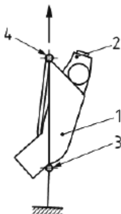
Рисунок 9 - Проверка прочности спасательных петель класса А статической нагрузкой
