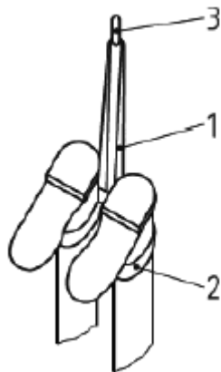
1 - спасательная петля; 2 - основная лямка; 3 - элемент крепления
