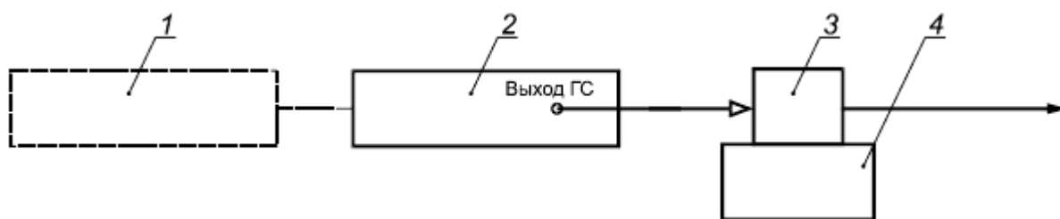
Рисунок Б.2 - Газовая схема для подачи ГС на газоанализаторы с диффузионным отбором пробы (а - для генераторов или калибраторов без выхода сброса излишков ГС, б - для генераторов или калибраторов с выходом сброса излишков ГС)
