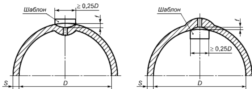
б) Совместный увод кромок (угловатость) в предельных швах
