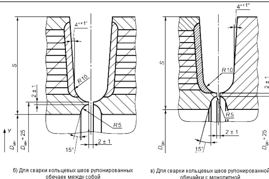
Рисунок 5 - Конструктивные элементы разделки кромок под наплавку торцов и автоматическую сварку кольцевых швов
