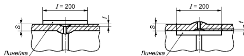
б) Совместный увод кромок (угловатость) в предельных швах
