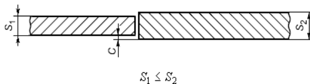
а) Смещение кромок
